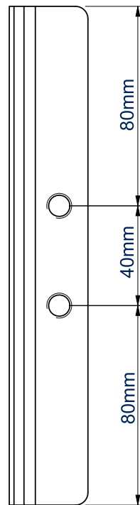
VUE LATÉRALE
