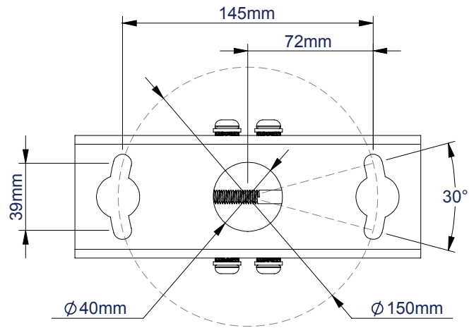
VUE TOP
