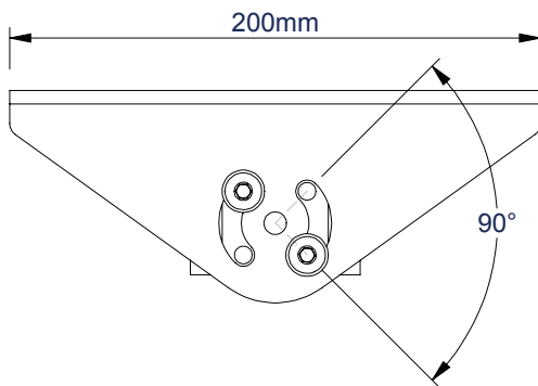
VUE LATÉRALE
