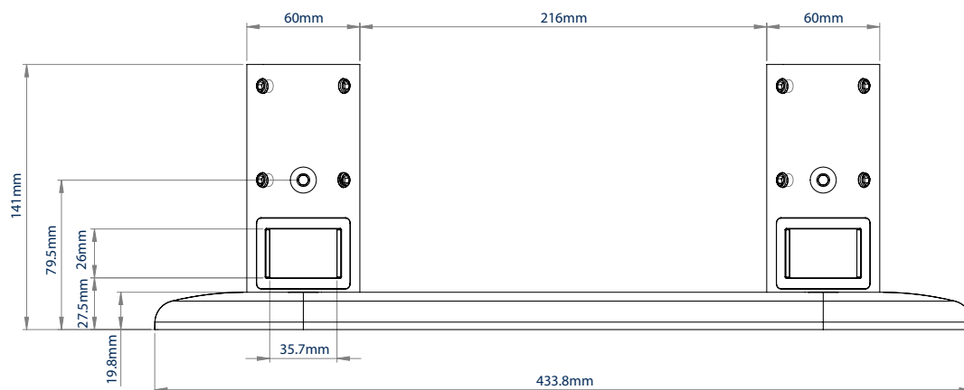
CÔTÉ VUE AVEC PLAQUE DE RECouvreMENT
