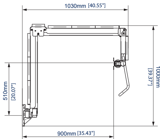
VUE LATÉRALE
