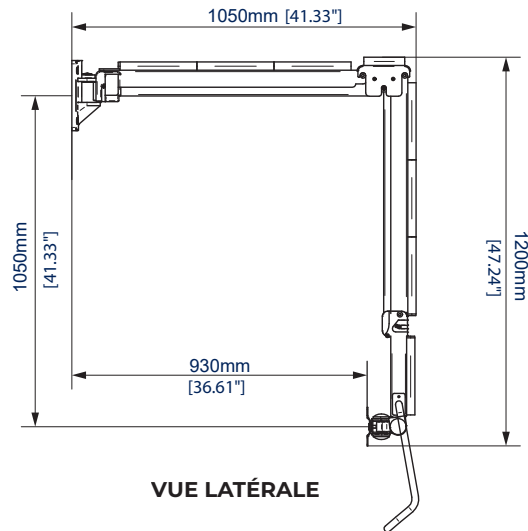
VUE LATÉRALE - EXTENSION MAXIMALE
