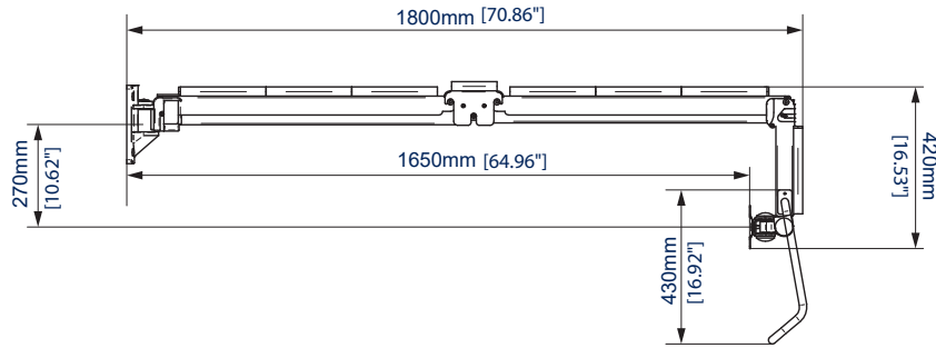
VUE LATÉRALE - EXTENSION MAXIMALE
