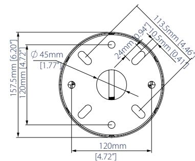
PLAQUE DE PLAFOND - VUE DE DESSUS
