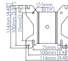
PLAQUE D'INTERFACE - VUE DE FACE
