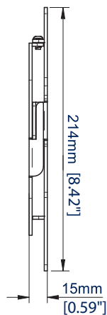
VUE LATÉRALE PLAQUE MURALE & PLAQUE D'INTERFACE
