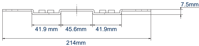
VUE LATÉRALE
