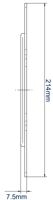
VUE LATÉRALE
