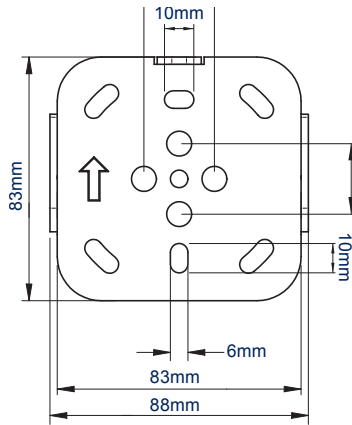
VUE DE FACE PLAQUE MURALE
