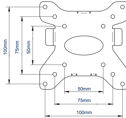
VUE DE FACE PLAQUE D'INTERFACE
