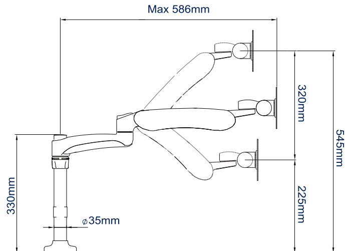
VUE LATÉRALE
