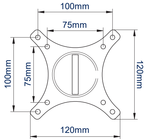
PLAQUE D'INTERFACE
