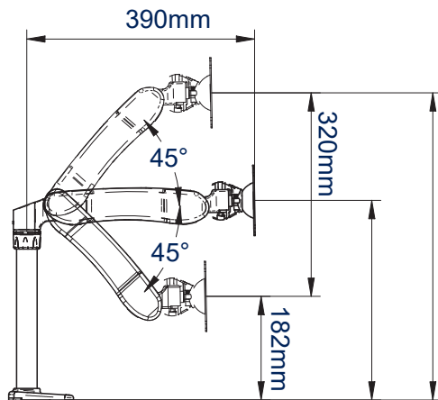
VUE LATÉRALE
