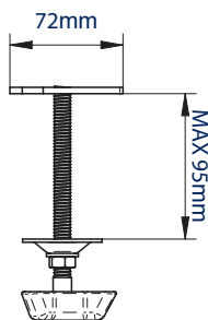
VUE LATÉRALE CÉILLET
