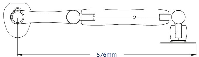
HAUT VUE - EXTENSION MAXIMALE
