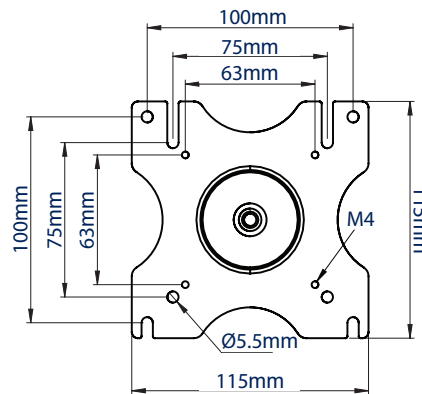
VUE DE FACE INTERFACE
