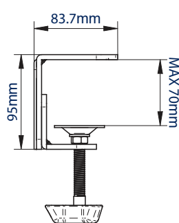
VUE LATÉRALE PINCE DE BUREAU
