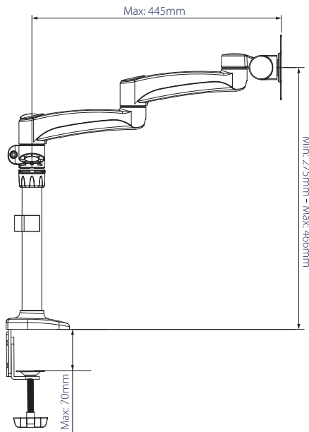
VUE LATÉRALE
