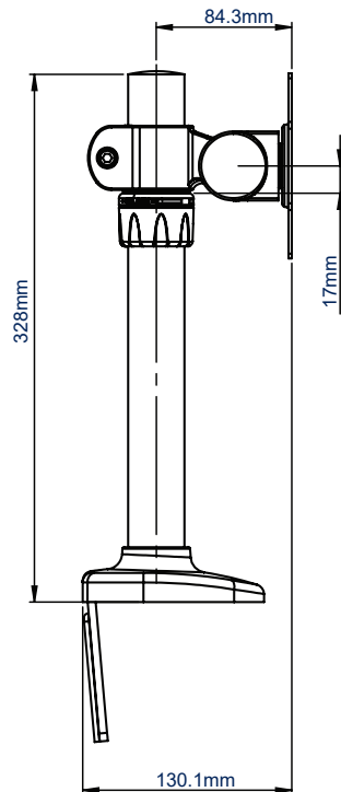
VUE LATÉRALE
