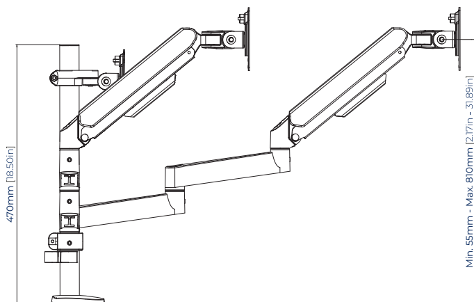
VUE LATÉRALE
