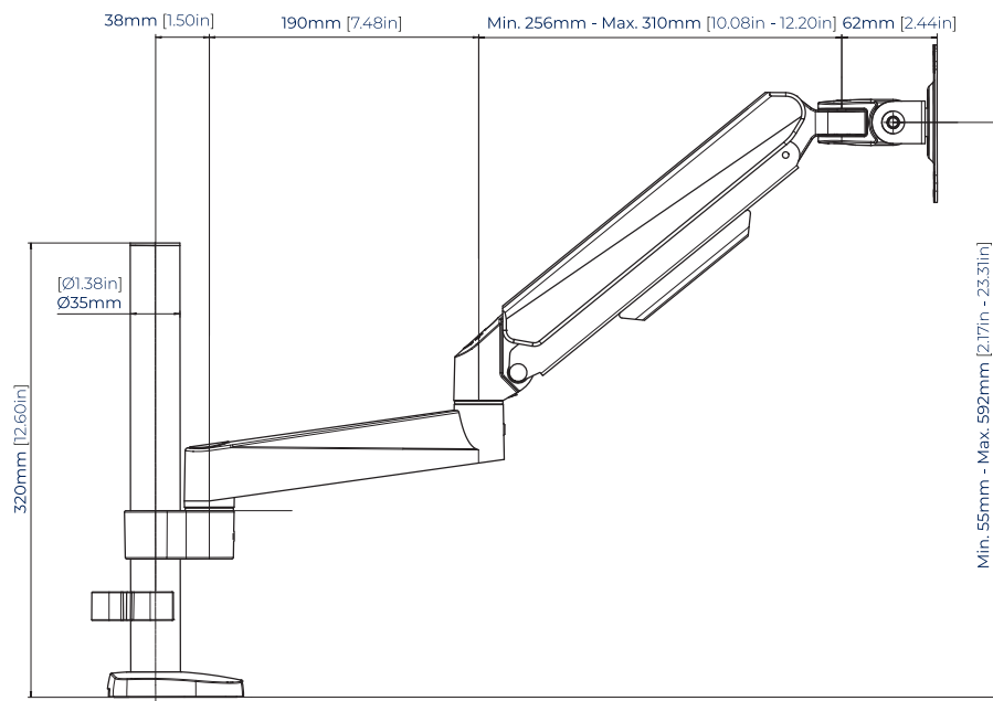
VUE LATÉRALE
