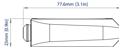
VUE DE CÔTÉ AVEC PLAQUE DE RECOUVREMENT
