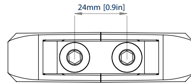
VUE DE FACE SANS PLAQUE DE RECOUVREMENT
