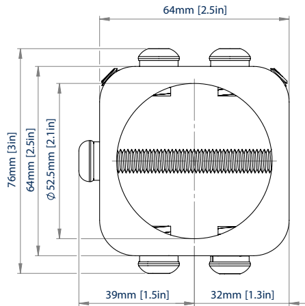
VUE DE DESSUS SANS PLAQUE DE COUVERTURE
