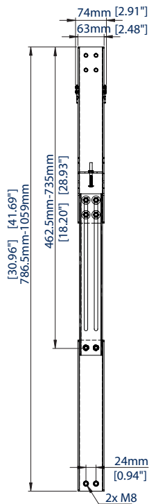
VUE DE FACE RAIL INFÉRIEUR ETENDU
