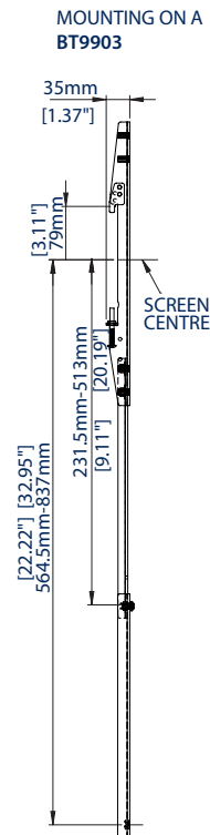
VUE LATÉRALE EN BAS DE L'ÉCRAN
