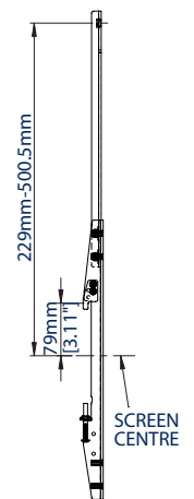
VUE LATÉRALE EN BAS DE L'ÉCRAN
