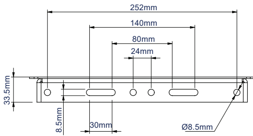
VUE ARRIÈRE
