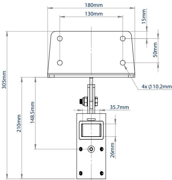
VUE ARRIÈRE
