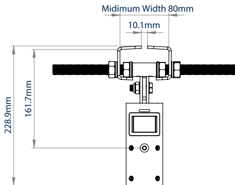
VUE DE FACE LARGEUR MINIMALE
