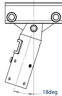
RÉGLAGE DE L'INCLINAISON 18 DEGRÉS
