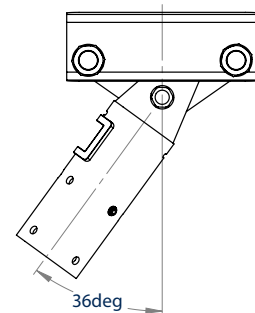
RÉGLAGE DE L'INCLINAISON 36 DEGRÉS (MAXIMUM)
