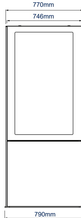
VUE ARRIÈRE
