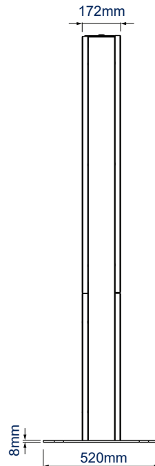
VUE LATÉRALE
