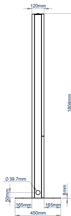
VUE LATÉRALE
