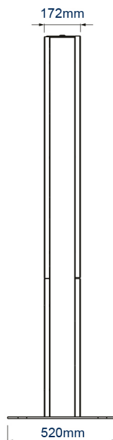
VUE LATÉRALE
