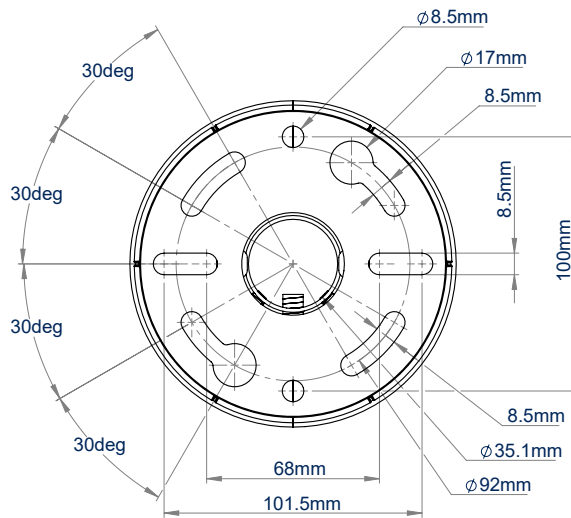
MONTAGE AU PLAFOND VUE DE DESSUS
