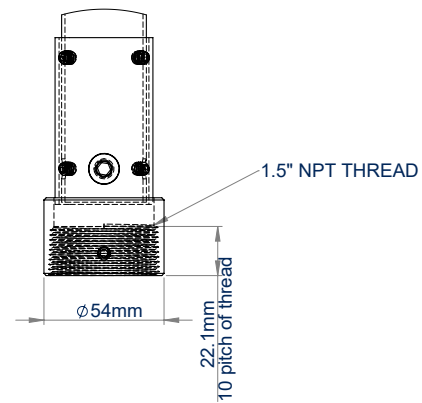
ADAPTATEUR NPT VUE DE FACE
