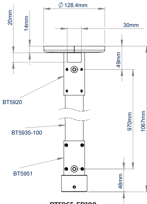
BT5965-FD100 VUE DE FACE
