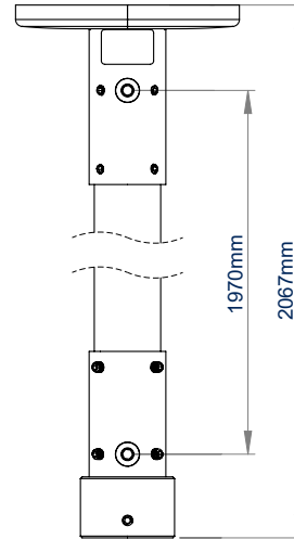
BT5965-FD200 VUE DE FACE
