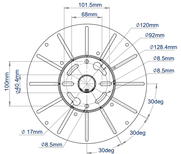
PLAQUE DE PLAFOND VUE DE DESSUS
