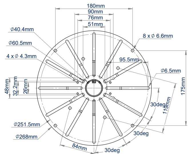
SUPPORT POUR CAMÉRA DE VIDÉOSURVEILLANCE VUE INFÉRIEURE
