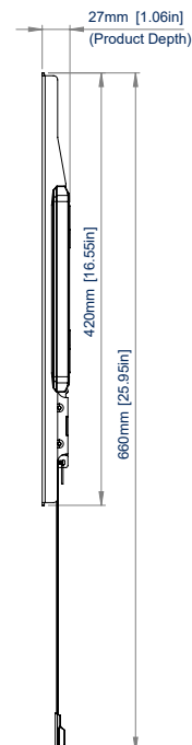
VUE LATÉRALE
