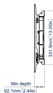
VUE LATÉRALE PRÈS DU MUR
