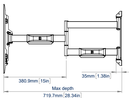
VUE LATÉRALE AVEC EXTENSION
