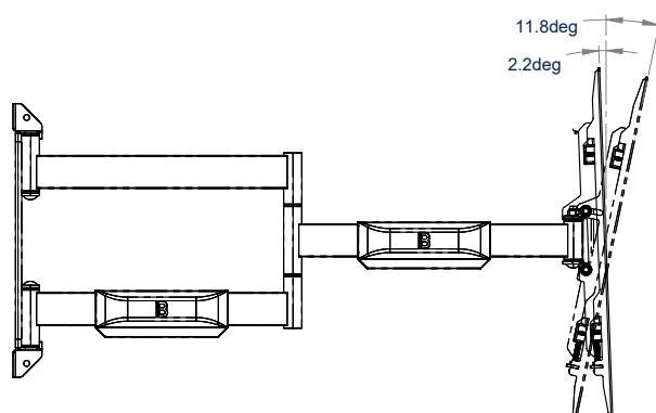
VUE LATÉRALE AVEC INCLINAISON
