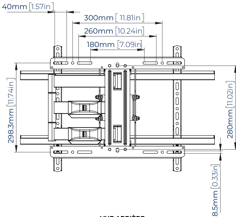
VUE ARRIÈRE
