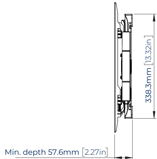
VUE LATÉRALE
