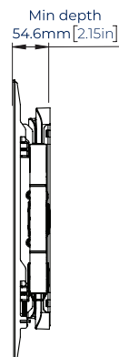
VUE LATÉRALE
