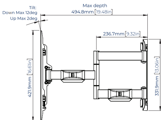
VUE LATÉRALE AVEC EXTENSION
