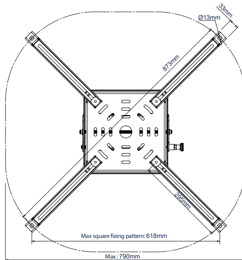
INTERFACE AVEC PIEDS D'EXTENSION LONGS ET PIEDS D'EXTENSION COURTS
