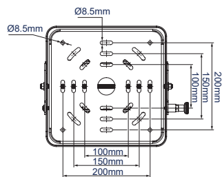
VUE DE DESSOUS PLAQUE D'INTERFACE
