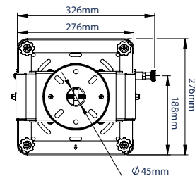
VUE DE DESSUS AVEC PLAQUE DE PLAFOND
