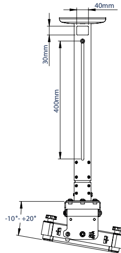
VUE LATÉRALE AVEC INTERFACE TILT
