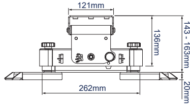
VUE LATÉRALE AVEC PIEDS D'EXTENSION COURTS INCLUS
