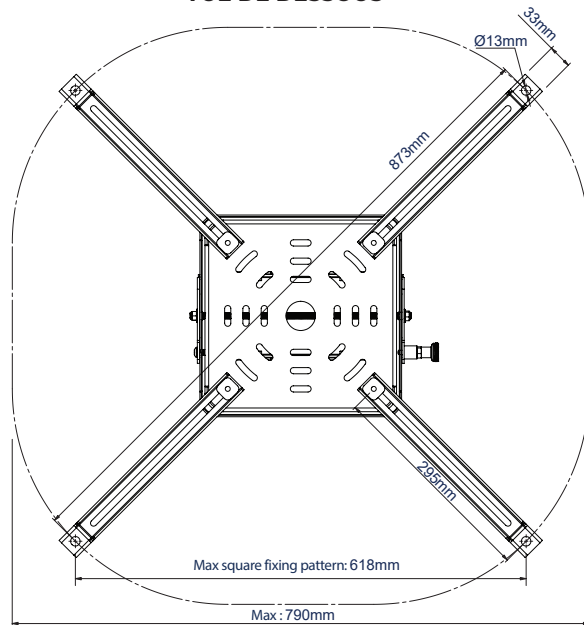
VUE DE DESSOUS AVEC PIEDS D'EXTENSION LONGS INCLUS
