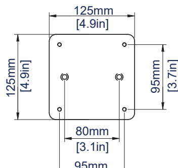
PLAQUE SUPÉRIEURE
