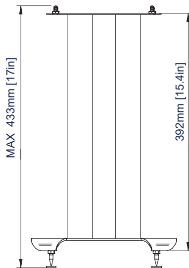
VUE AVANT
