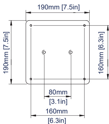
PLAQUE SUPÉRIEURE
