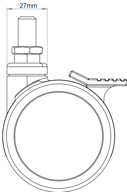
VUE LATÉRALE
