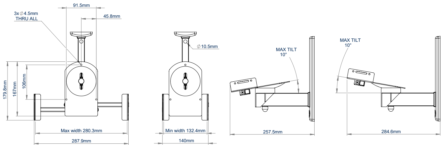
VUE TOP
