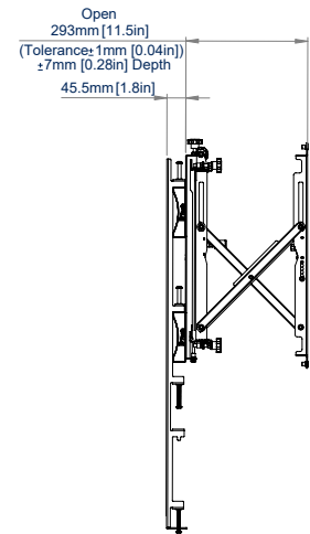
VUE LATÉRALE
