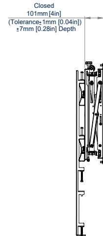
VUE LATÉRALE
