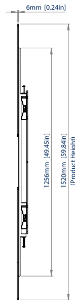
VUE LATÉRALE
