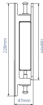
VUE LATÉRALE
