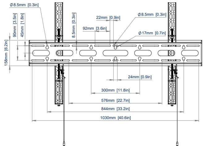
VUE ARRIÈRE
