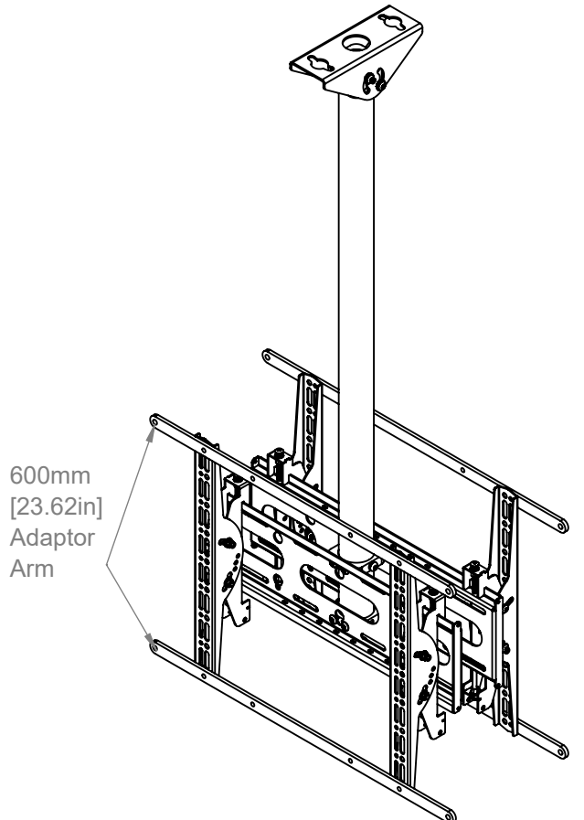
ISOMETRIC VIEW SCALE: 1 : 10
