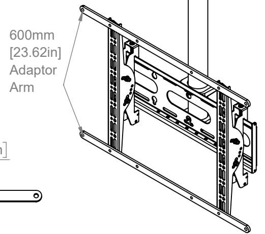
ISOMETRIC VIEW SCALE: 1 : 10
