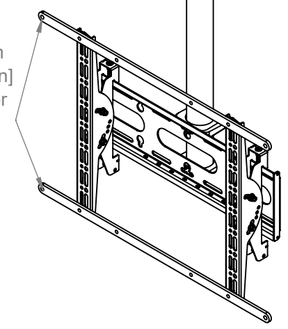
ISOMETRIC VIEW SCALE: 1 : 10
