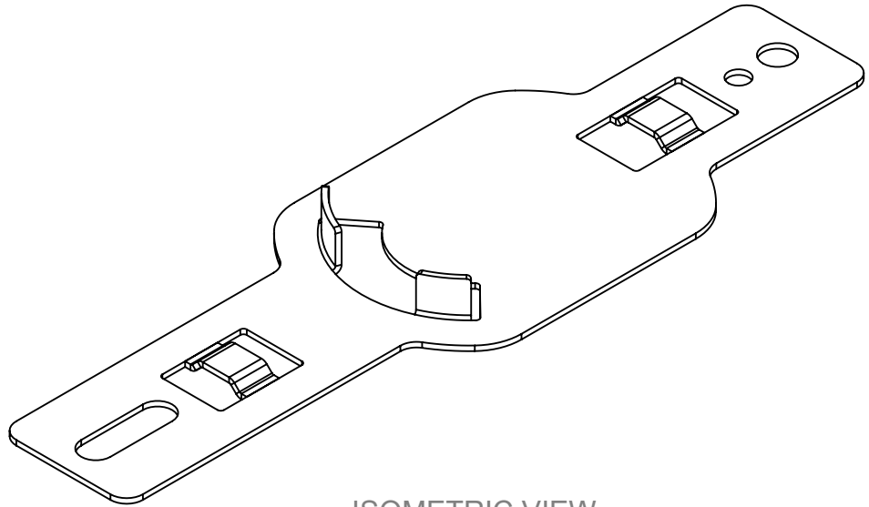
ISOMETRIC VIEW SCALE: 2 : 3
