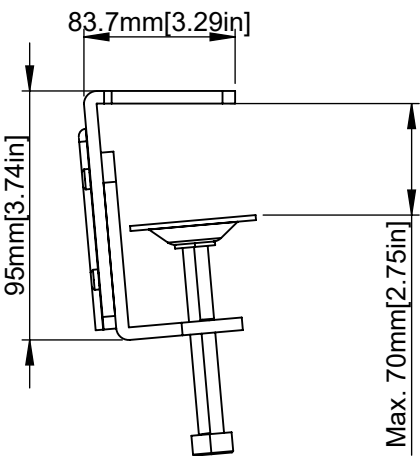
SCALE 1 : 3 Grommet Clamp
