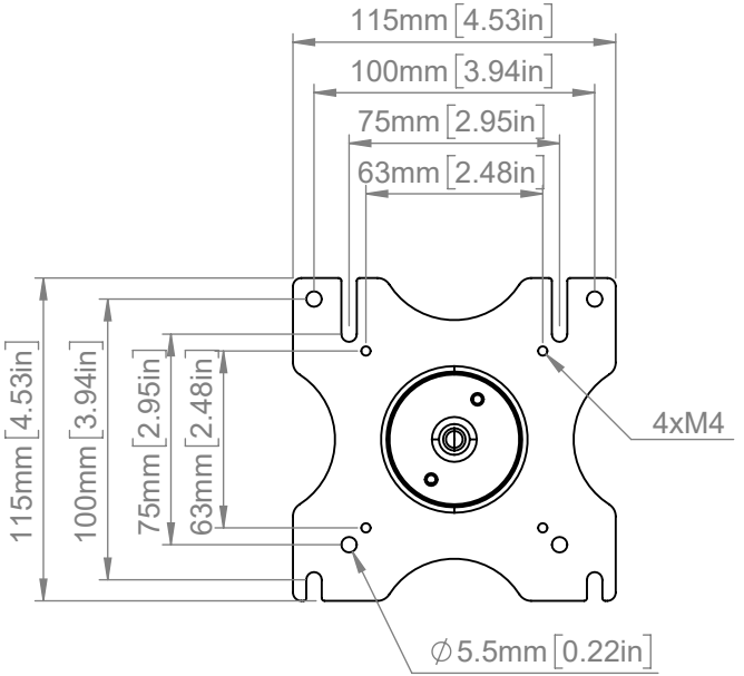
SCALE 1 : 3
