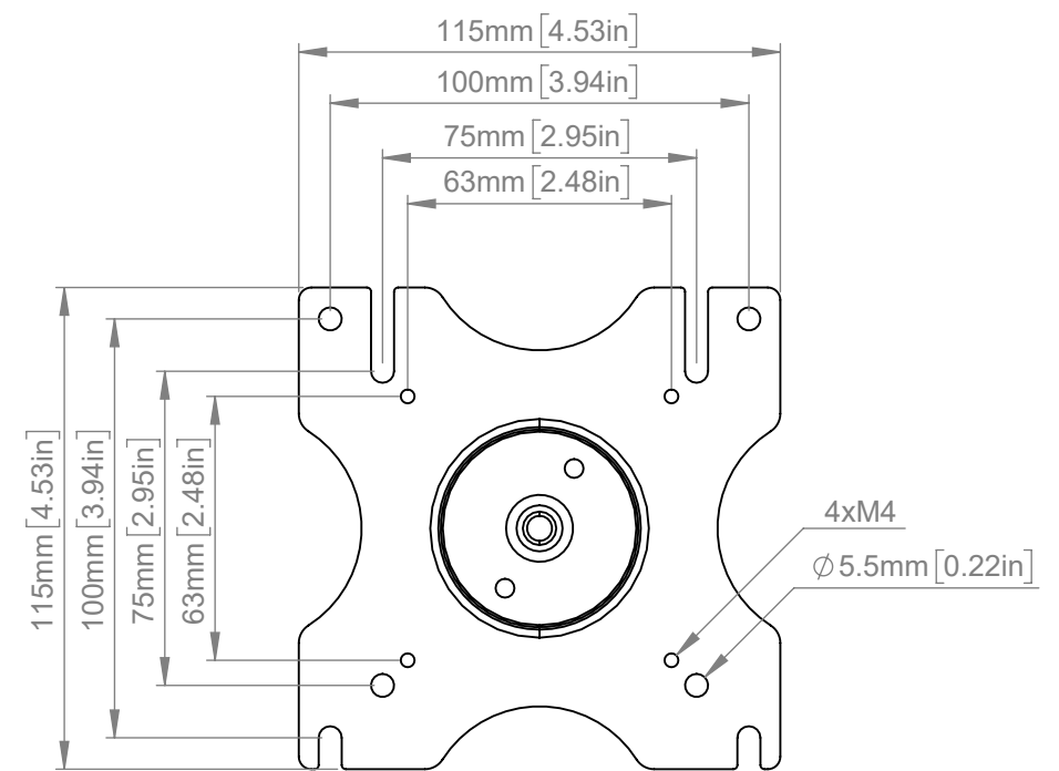
SCALE 1 : 2
