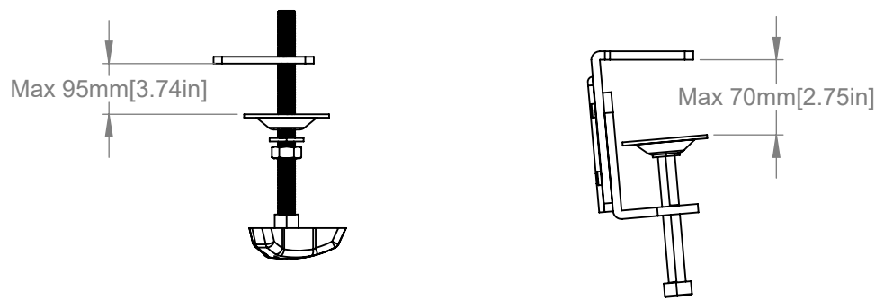
Grommet Clamp
