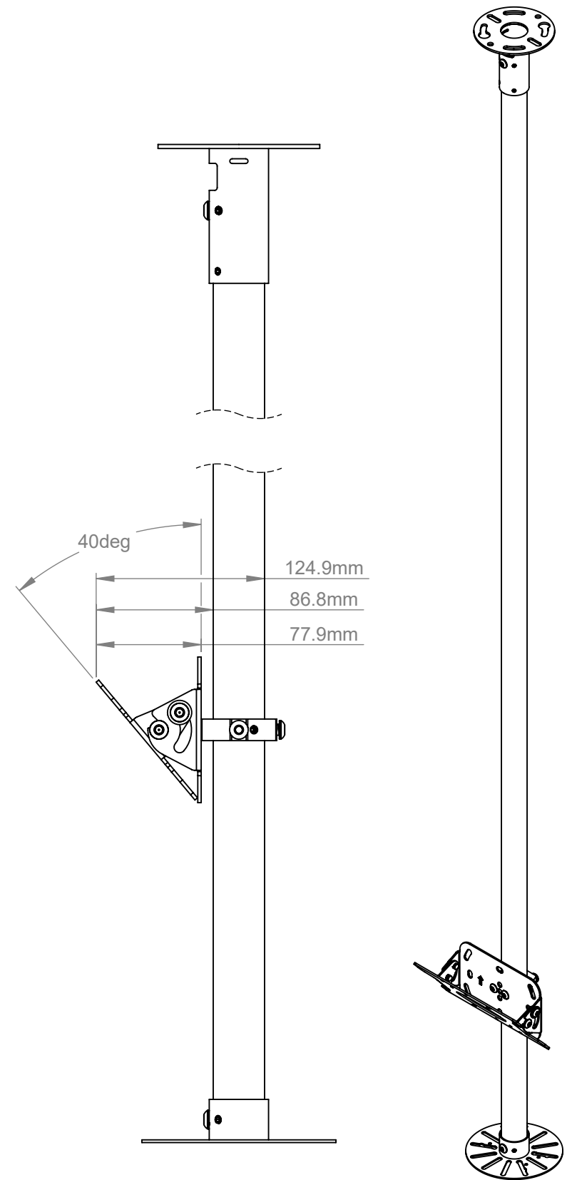
ISOMETRIC VIEW SCALE: 1 : 8
