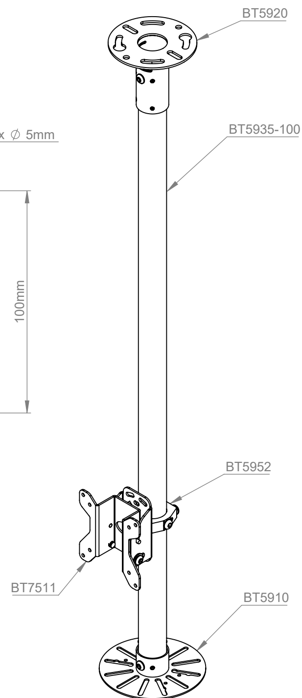
ISOMETRIC VIEW SCALE: 1 : 5
