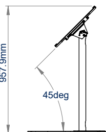
45° TILT
