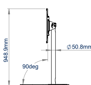
90° TILT
