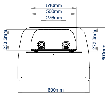
STAND BASE
